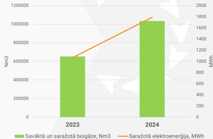
Saražotā biogāze un elektroenerģija AEC "Daibe"
